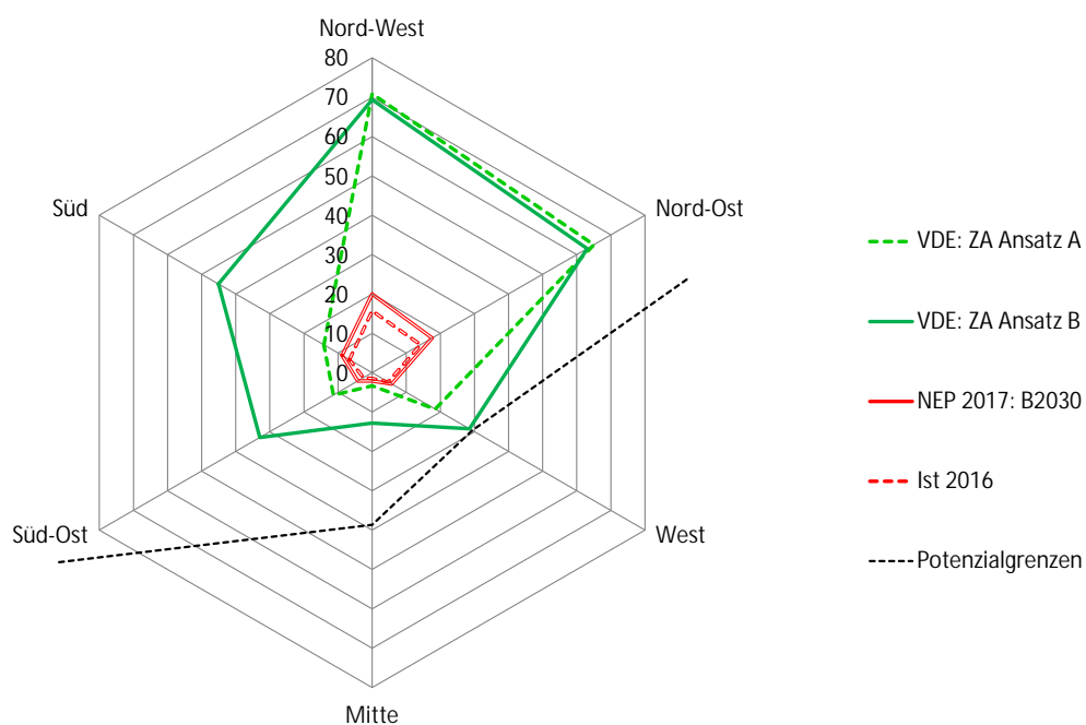
Abbildung 4-3: Regionalisierungsansätze Wind, Ausblick
