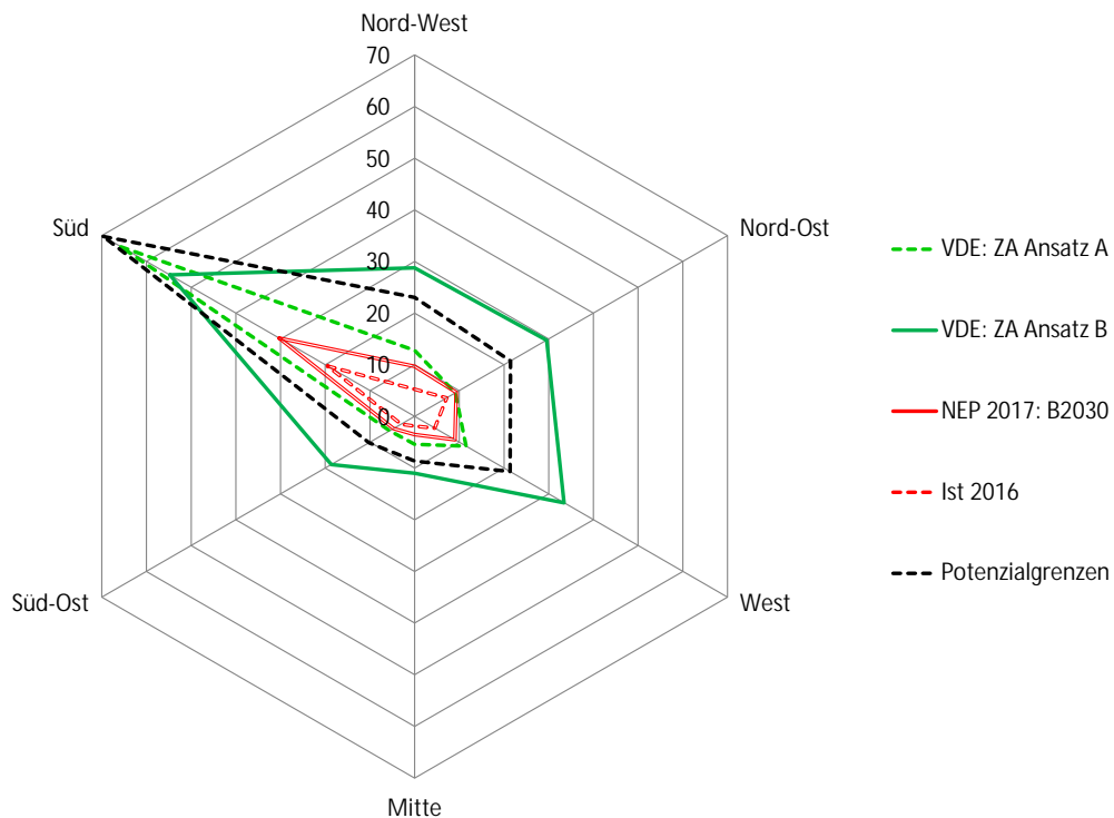
Abbildung 4-6: Regionalisierungsansätze Fotovoltaik, Ausblick
