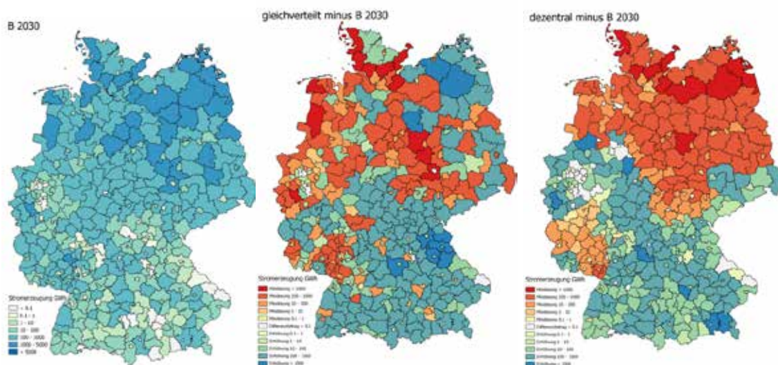
Abbildung 3-5: Windstromerzeugung im Szenario NEP B 2030 (links) und ihre Veränderung in den Szenarien „dezentral“ (Mitte) und „gleichverteilt“ (rechts)
