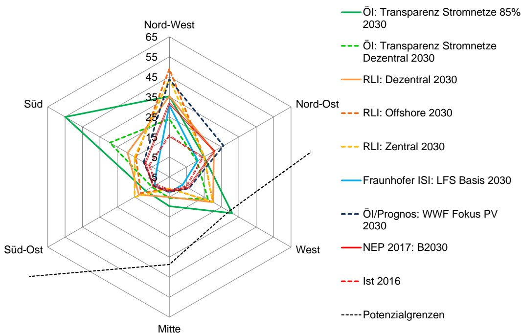
Abbildung 4-1: Regionalisierungsansätze On- und Offshore-Wind, 2030
