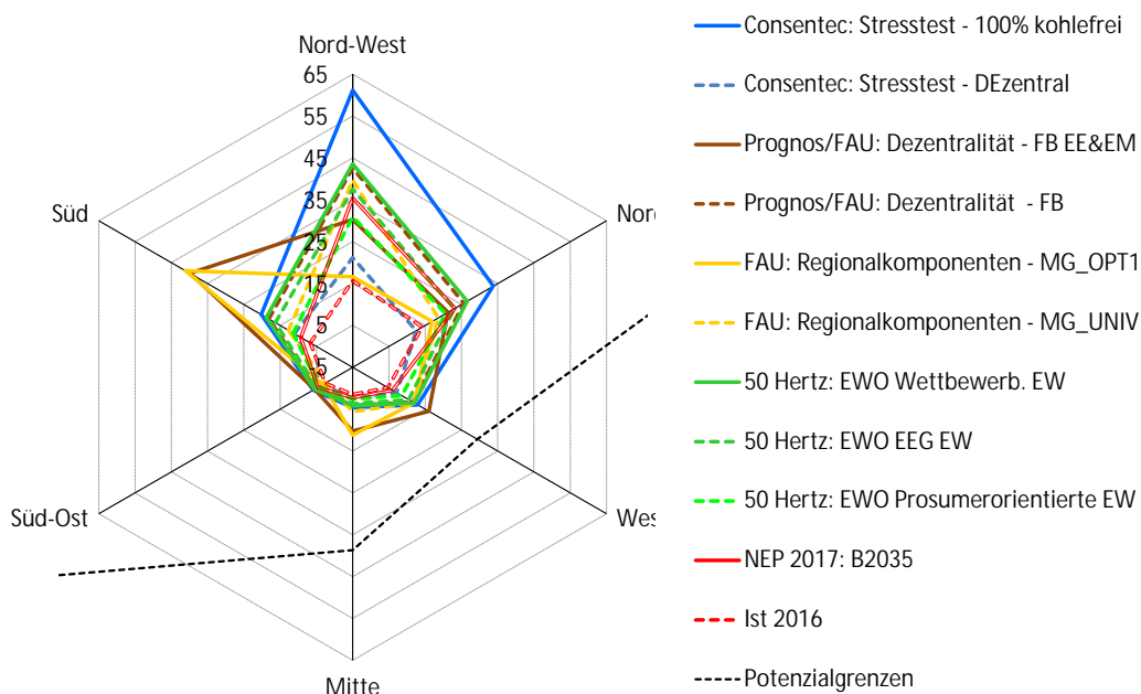
Abbildung 4-2: Regionalisierungsansätze On- und Offshore-Wind, 2035
