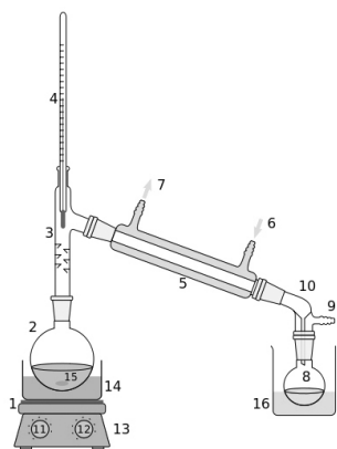
Abbildung V.4: Schemazeichnung einer Destillationsapparatur
